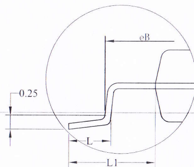
DETAIL: F
